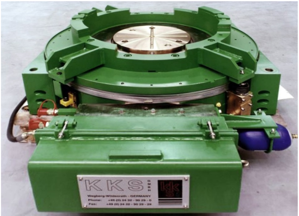
Anstellzylinder für eine Grobblechstraße in Ungarn
