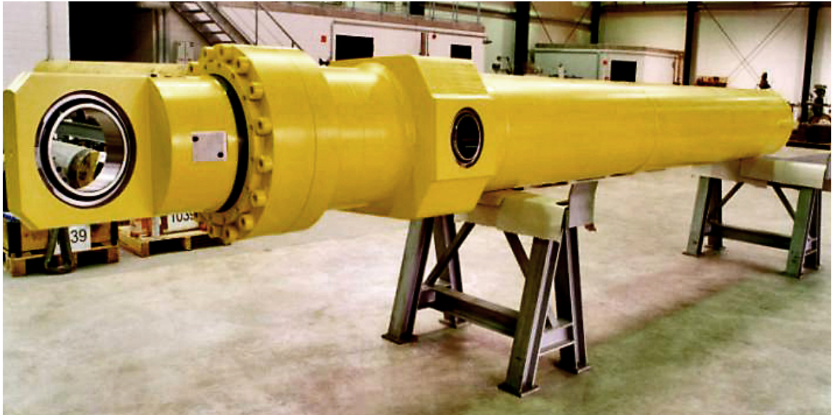
Ofenkipfzylinder für Aluminiumschmelzöfen
