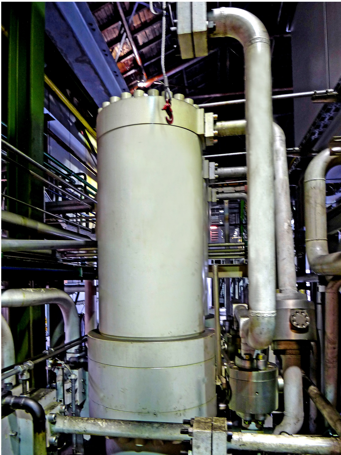
Druckübersetzer beim Kunden eingebaut
