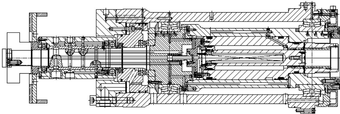
Arbeitsspindel für eine Reibschweißmaschine
