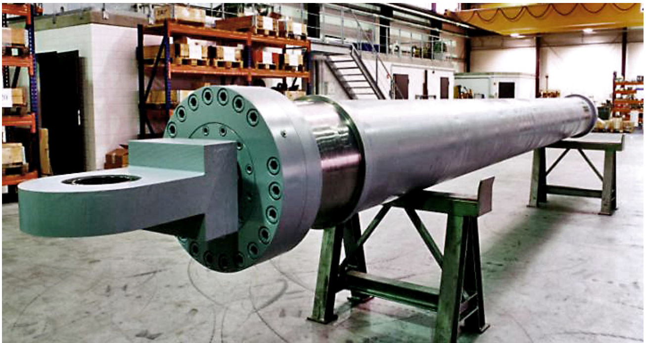
Verschiebezylinder 12m Hub
