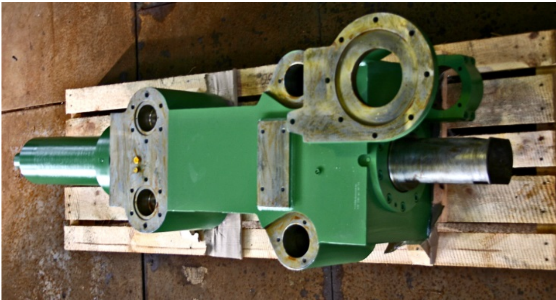
Sonderzylinder zum Einbau in eine Heftschweißmaschine
