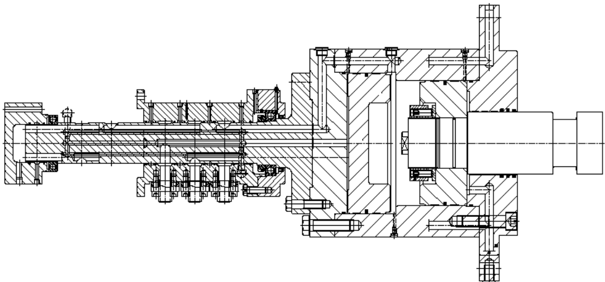
Zylinder mit Drehdurchführung
